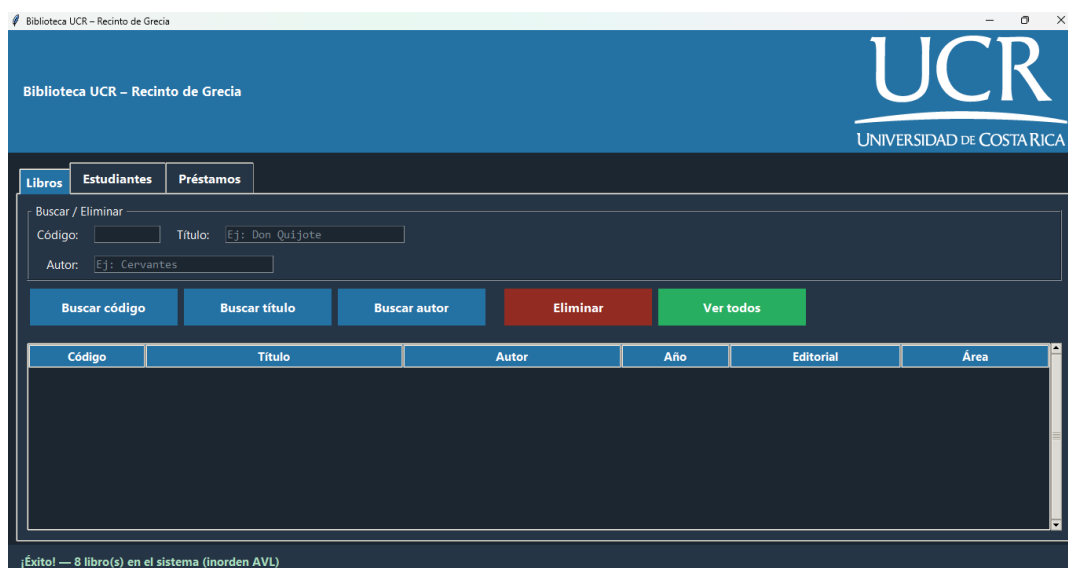
Figura 2: Pestaña Libros : formulario de búsqueda y tabla de resultados.
